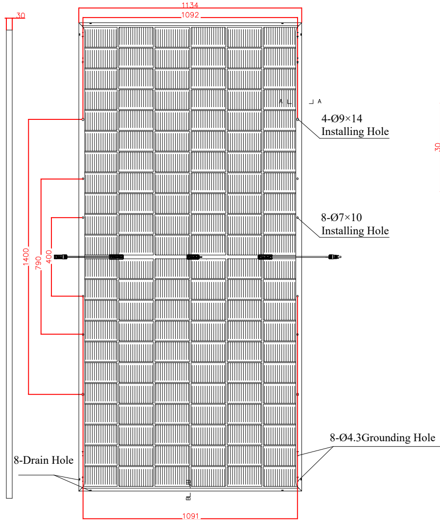
后视图
